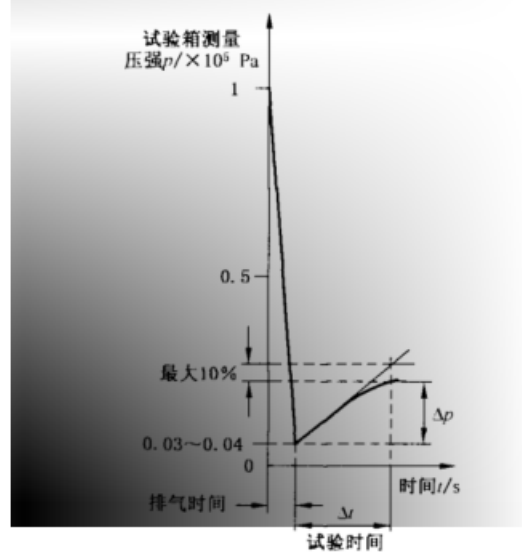
图 3 增压密封试验期间试验箱测量压强与测试时间的关系
