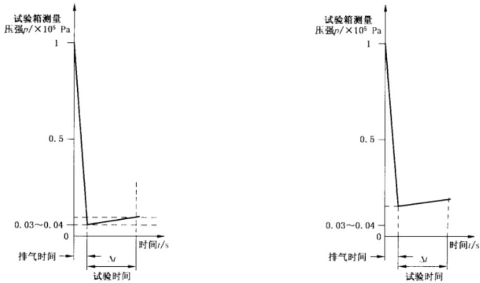
a) 紧闭装置,即漏率小于 10^{-4} \text{ Pa} \cdot \text{m}^3/\text{s} 或达到 10^{-5} \text{ Pa} \cdot \text{m}^3/\text{s} b) 大渗漏装置,即排气时间内达不到标定的低气压
