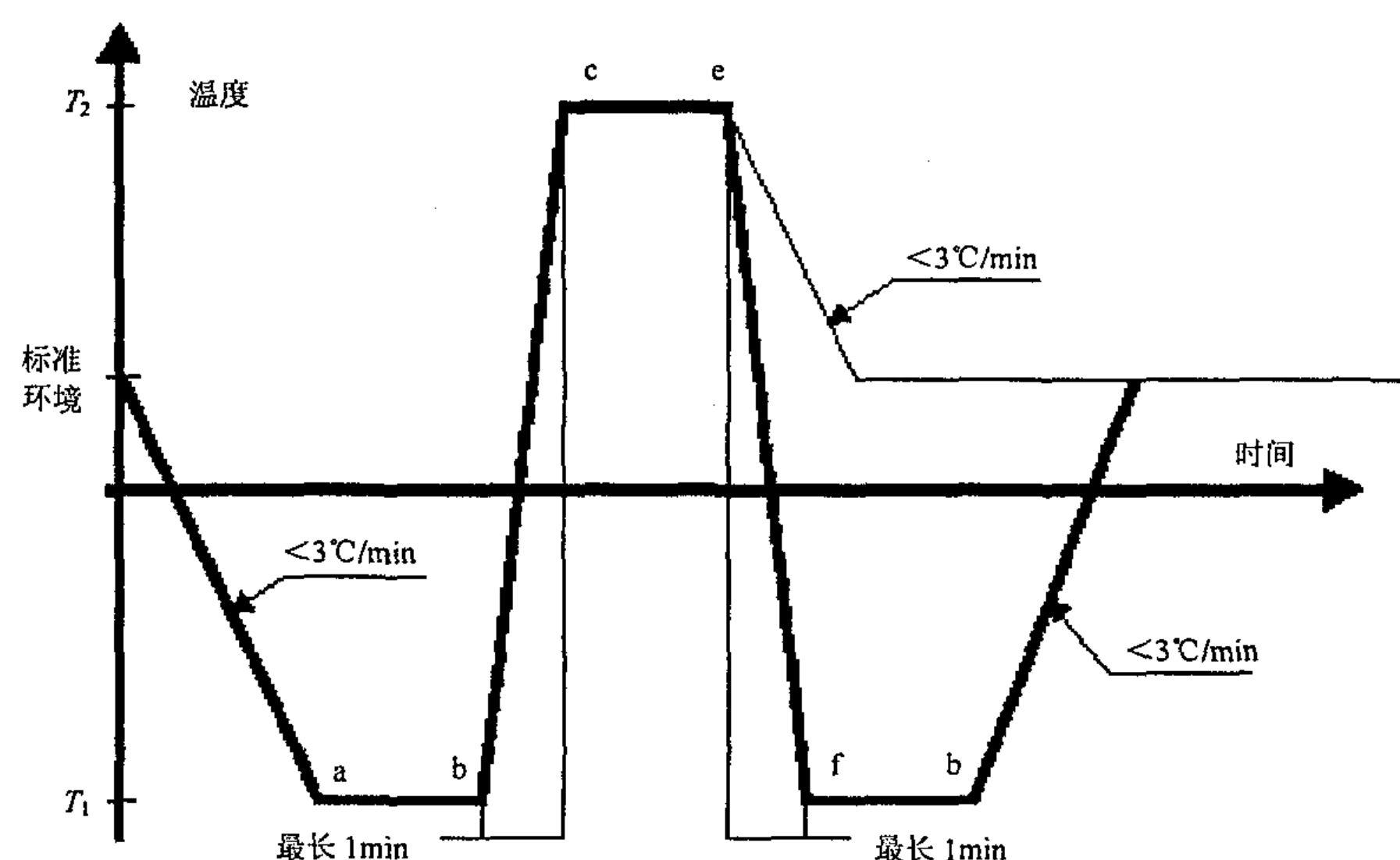
图 1 恒定极值温度冲击
