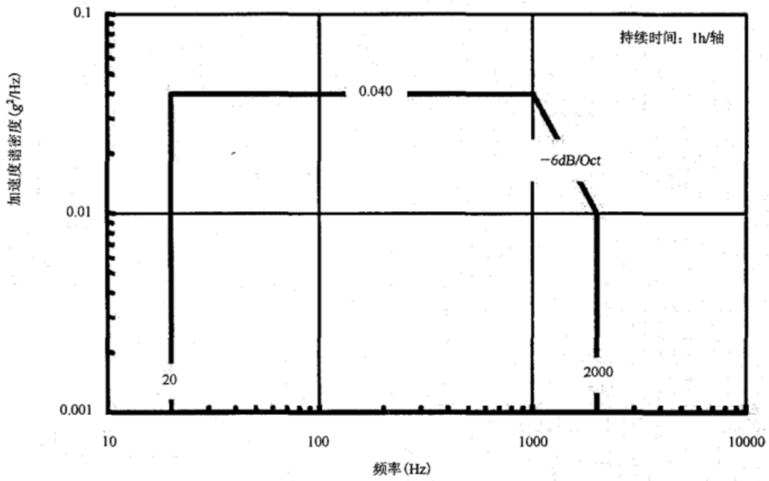
图 C.17 通用低限完整性振动试验环境
