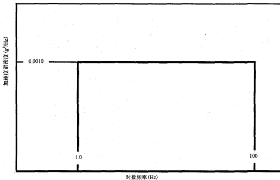
图 C.15 舰船随机振动环境
