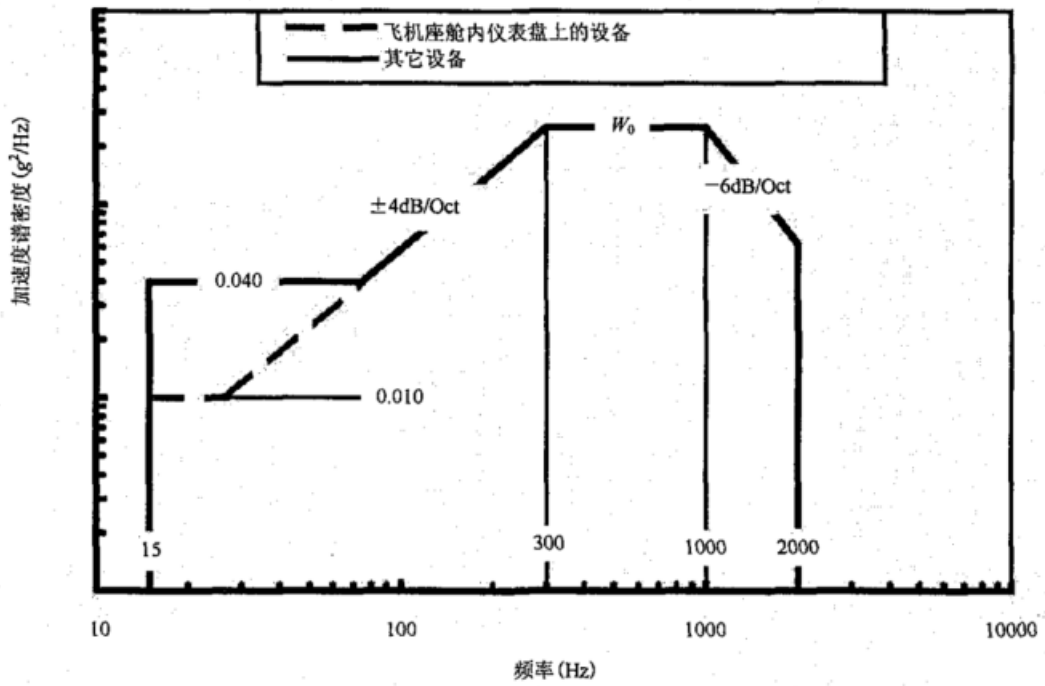
图 C.8 喷气式飞机振动环境
