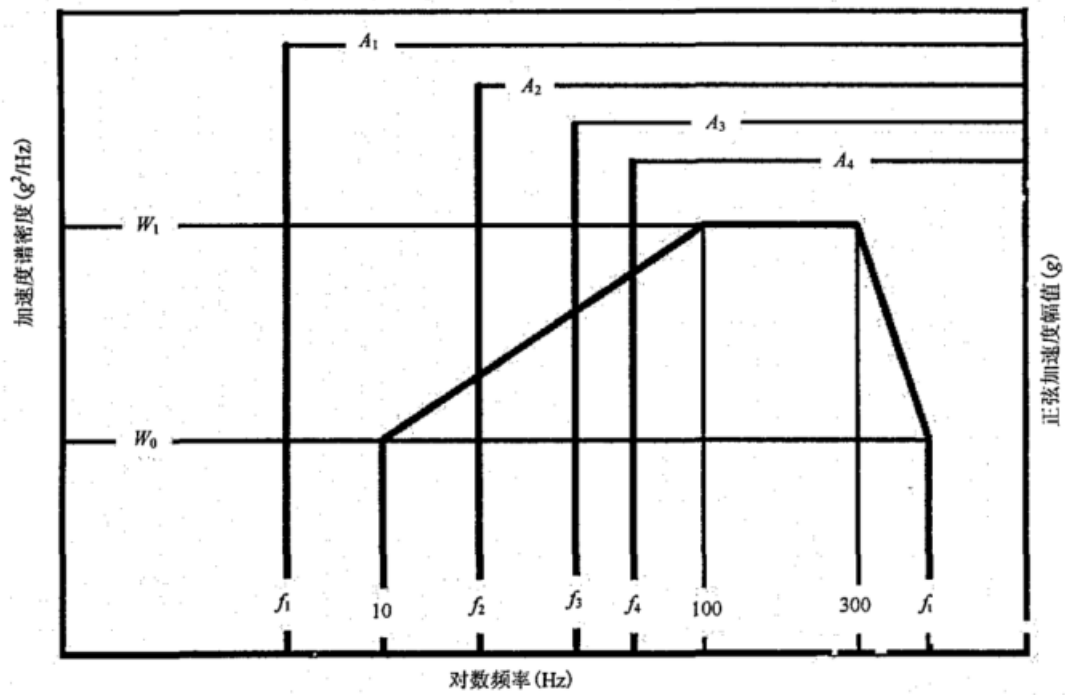
图 C.10 直升机振动环境
