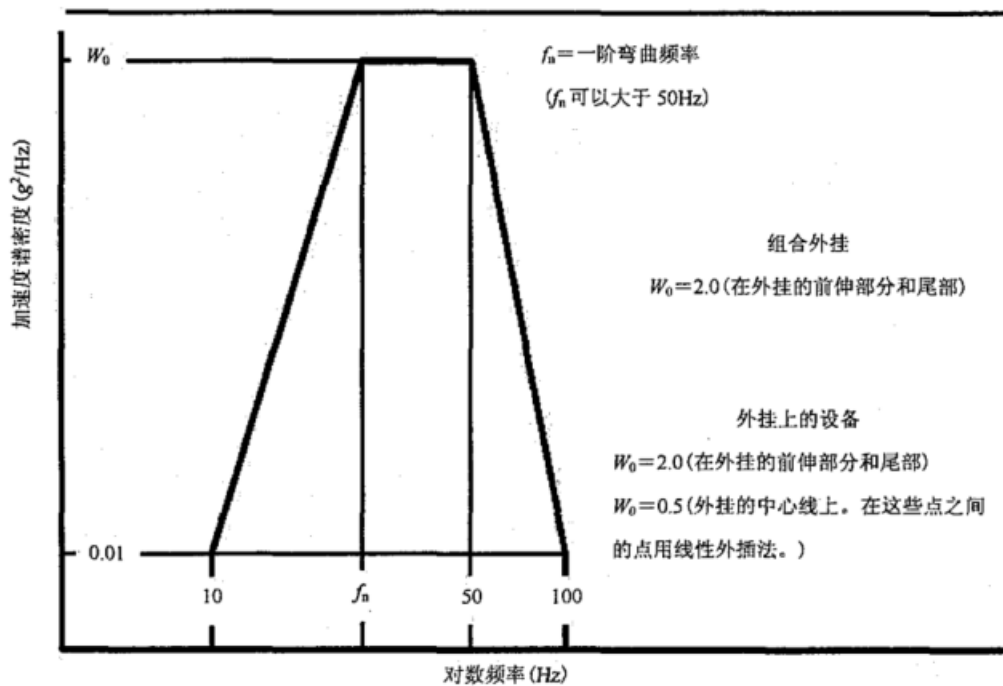
图 C.13 喷气式飞机外挂抖振响应
