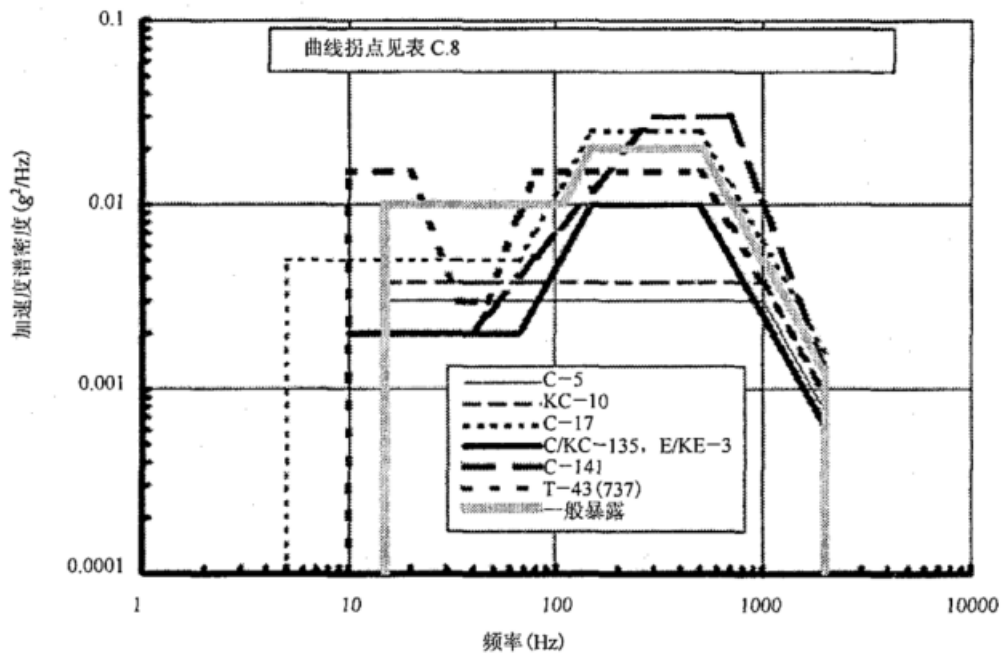
图 C.6 喷气式飞机货物振动环境
