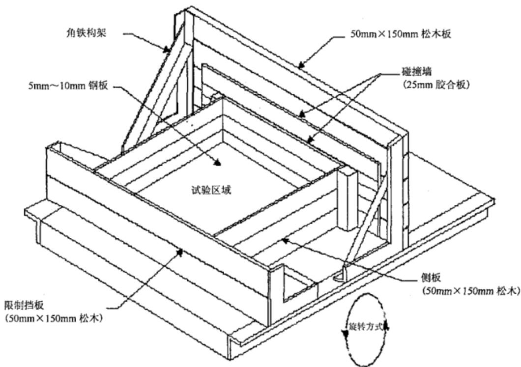
图 C.5 散货件货物试验装置
