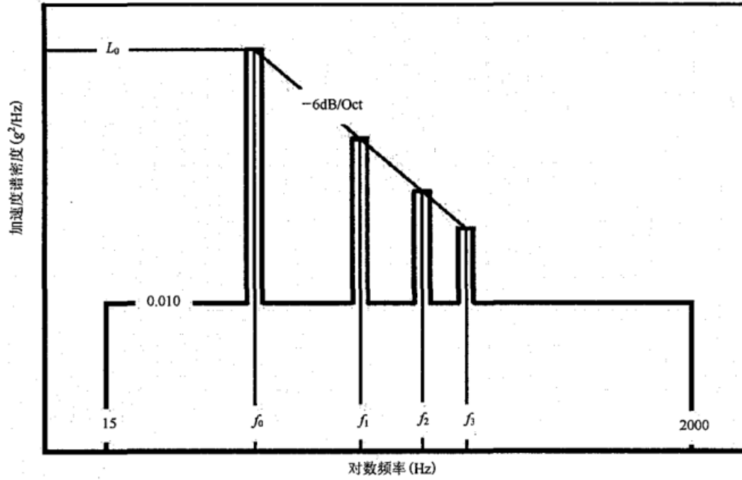
图 C.9 螺旋桨飞机振动环境
