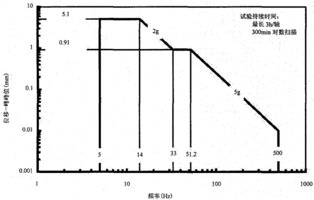
图 C.18 直升机低限完整性振动试验环境
