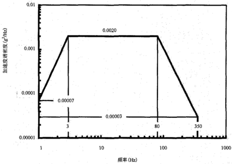
图 C.7 铁路货物振动环境
