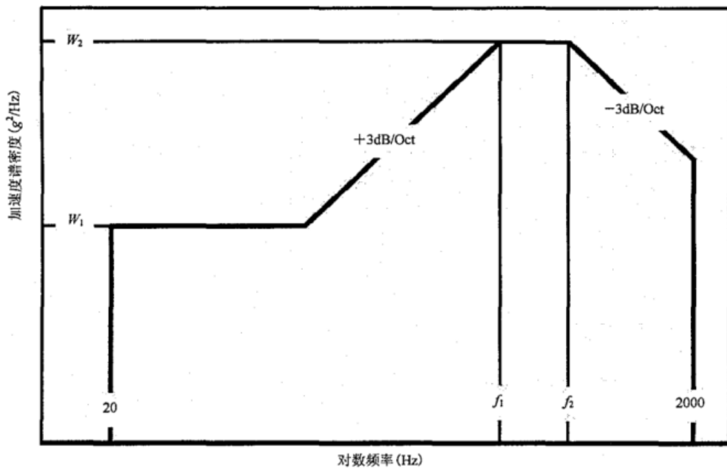
图 C.14 喷气式飞机外挂设备振动环境
