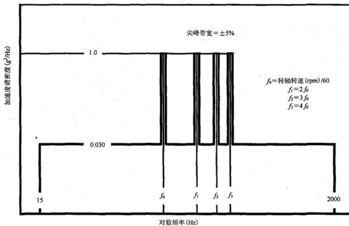
图 C.16 涡轮发动机振动环境
