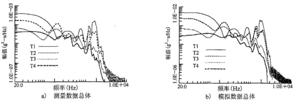
图 B. 8 短时能量谱密度函数估计(数据)
