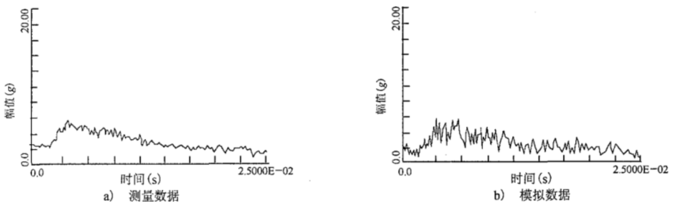
图 B.5 总体时变标准差估计
