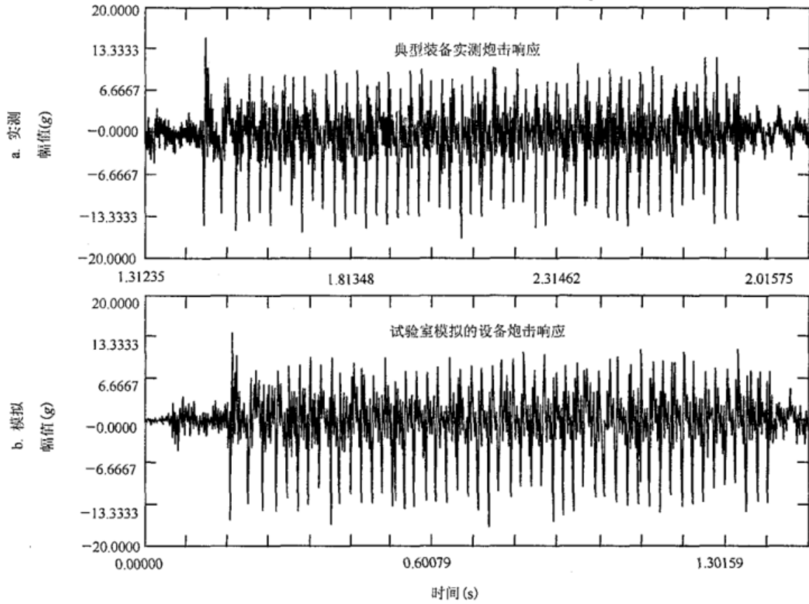
图 A. 7 装备实测炮击响应与实验室模拟的设备炮击响应的对比
