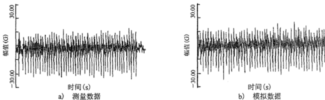
图 B. 1 50 发 30mm 炮击信号
