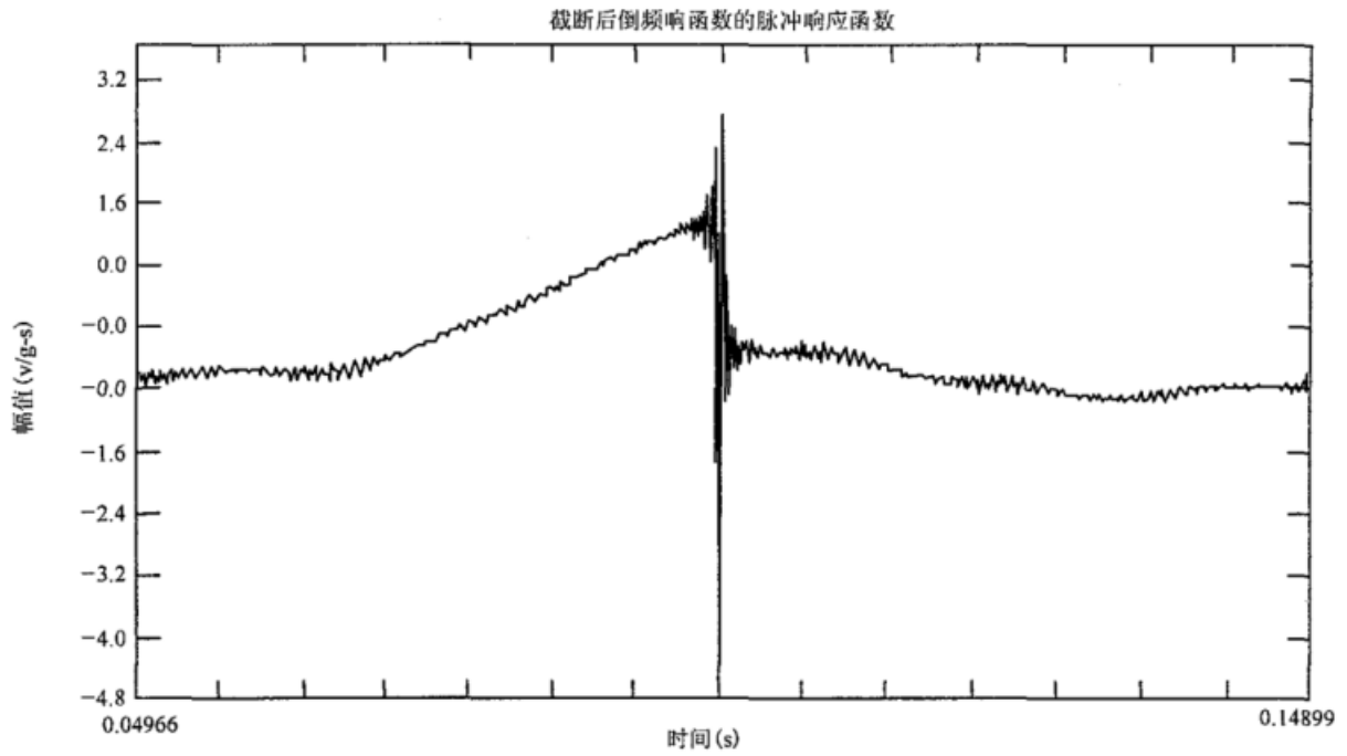
图 A. 5 脉冲响应函数
