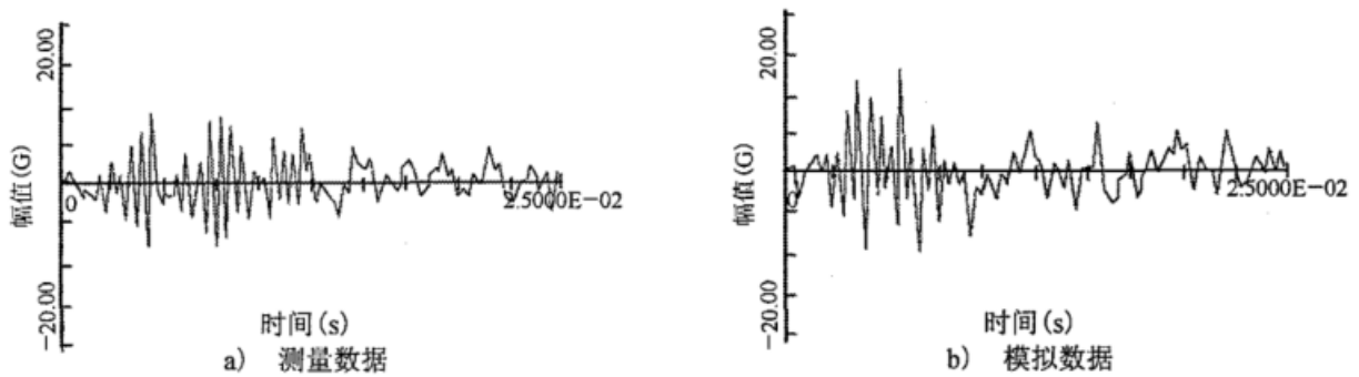
图 B.3 总体残余样本时间历程脉冲(第 37 脉冲)
