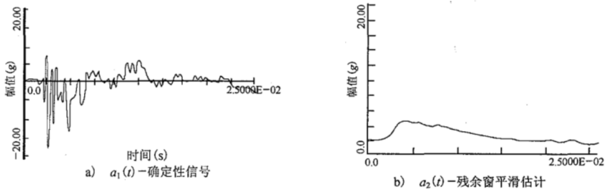
图 B. 10 非平稳模型确定性函数
