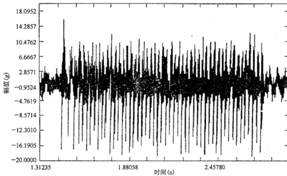
图 C. 1 数字化的测量数据
