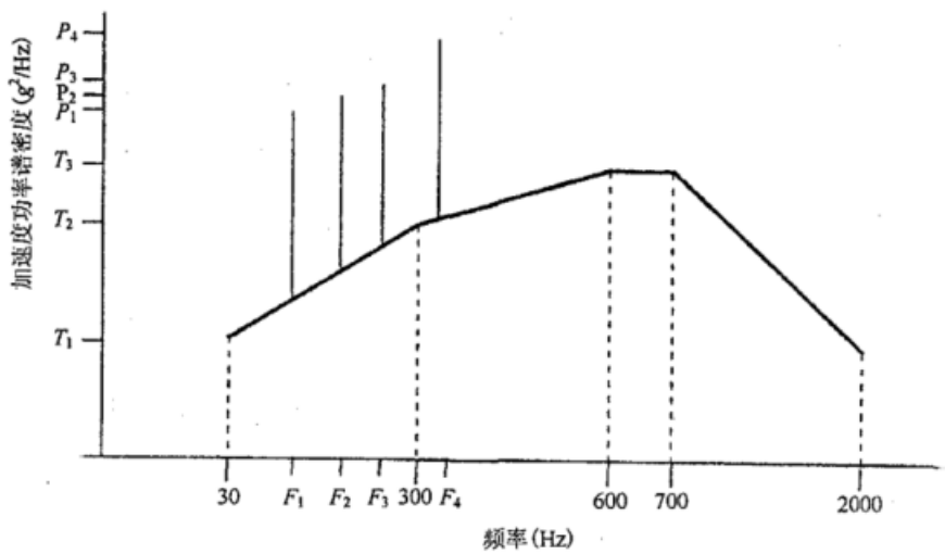
图 D. 1 通用的炮击诱发振动谱
