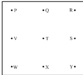
图 2 盐雾沉降率测量点布放位置示意图
