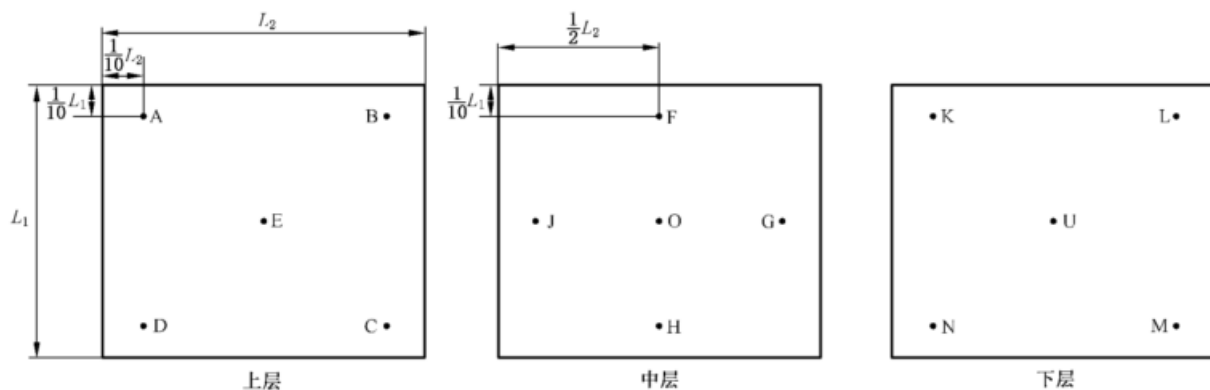
图 1 温度测量点布放位置示意图
