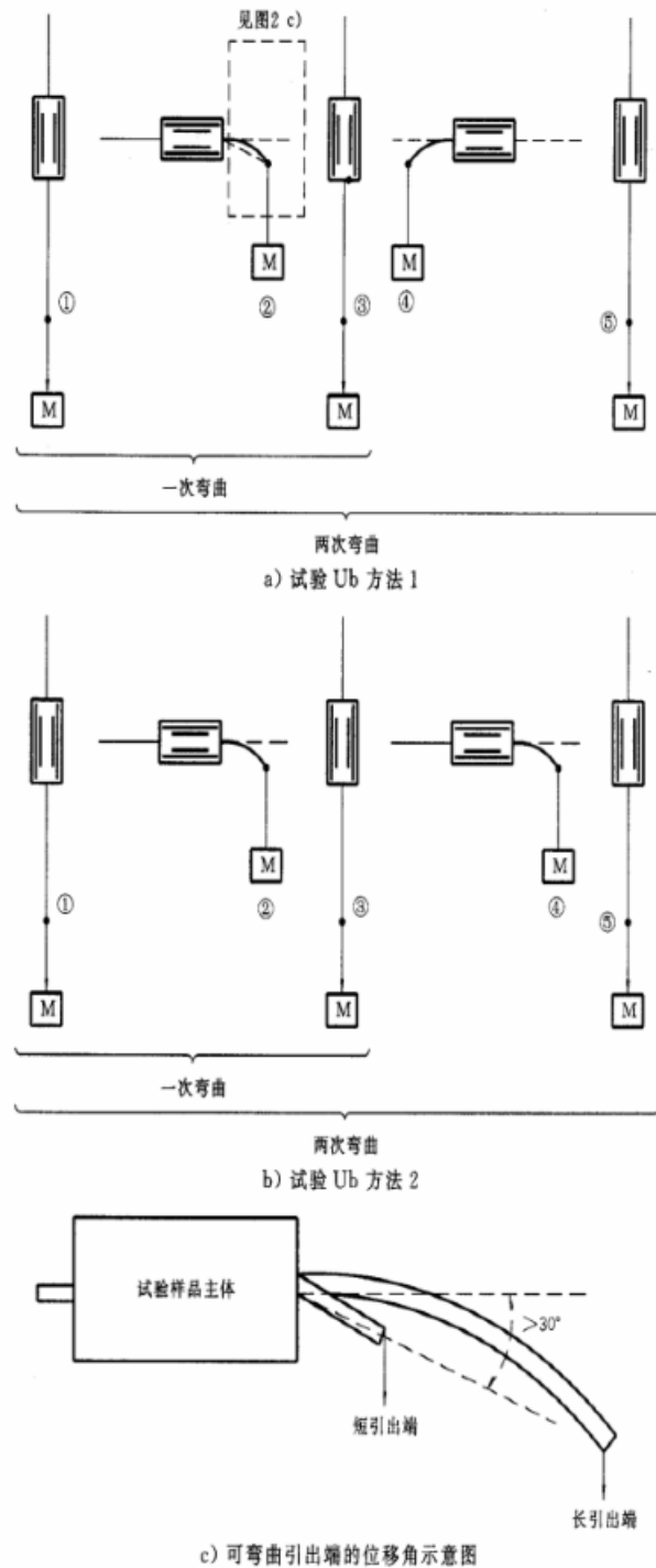
图 2 试验 Ub，弯曲试验的试验程序示意图(见 4.5.2.1~4.5.2.3)
