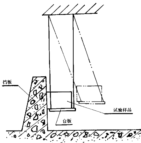
图 2 吊摆冲击试验机简图
