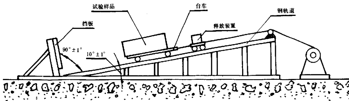
图 1 斜面冲击试验机简图
